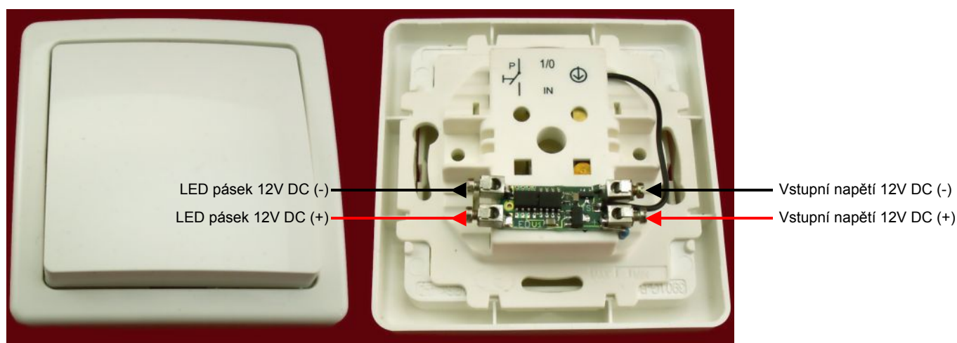
Obr. 1 - Zapojení vývodů stmívače
